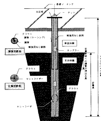
図1 高耐力マイクロパイルの概要図
