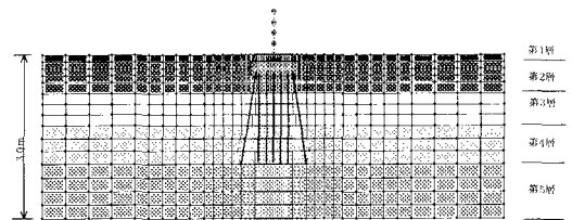
図2 解析メッシュ図
