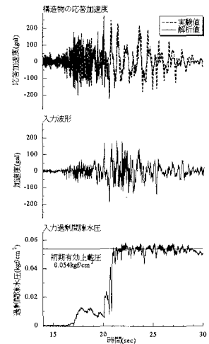
図3 応答加速度の時刻歴
