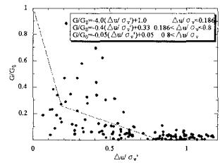
図2 G/G_0 \sim \Delta u/\sigma'_v の関係
