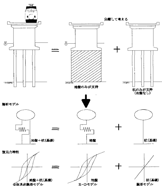
図1 解析モデル
