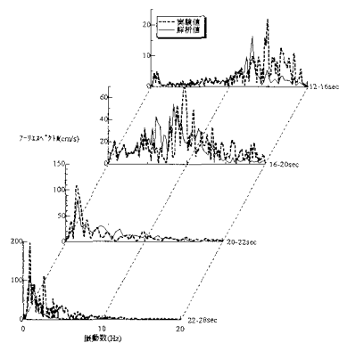
図4 ランニングスペクトル
