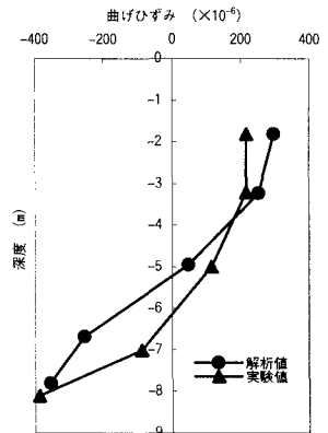
図2 シミュレーション解析結果：基礎杭の曲げひずみ分布
