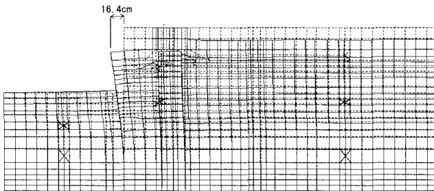
図3 シミュレーション解析結果：全体変形
