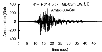
図 2 入力加振波
