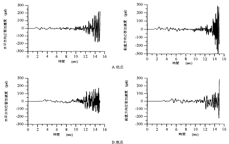
図-4 着目点の応答加速度時刻
