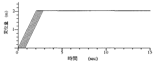
図-2 強制変位の条件
