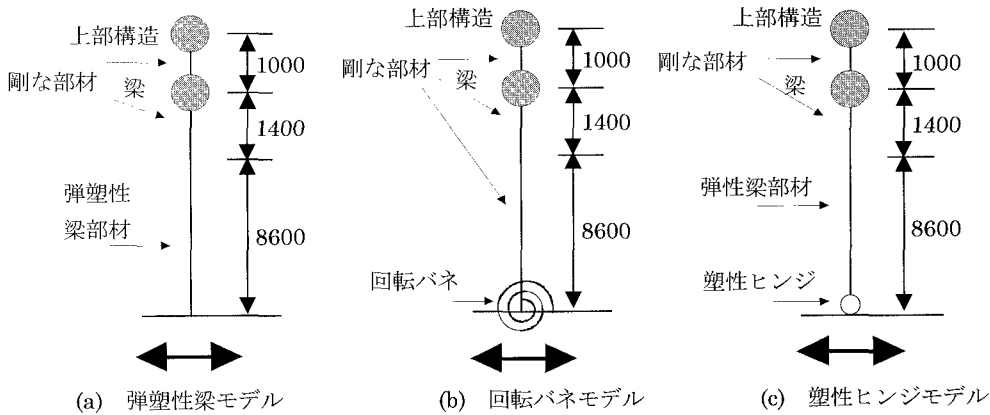
図 2 解析モデル
