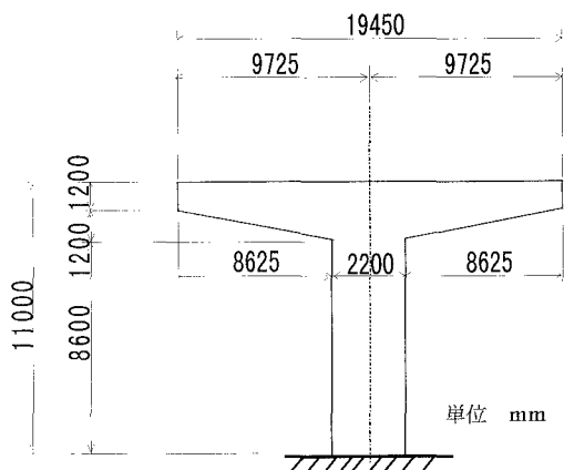
図 1 橋脚モデル
