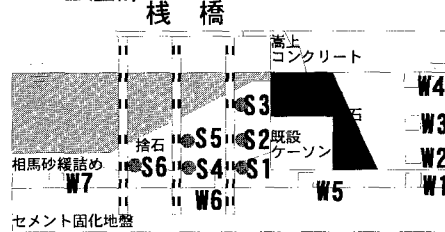
図-1 土圧計および間隙水圧計の設置位置
