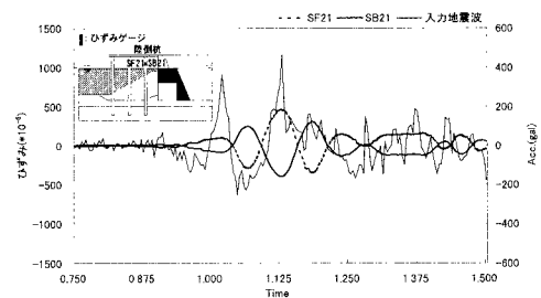
図-6 陸側杭のひずみの時刻歴 (CASE3)
