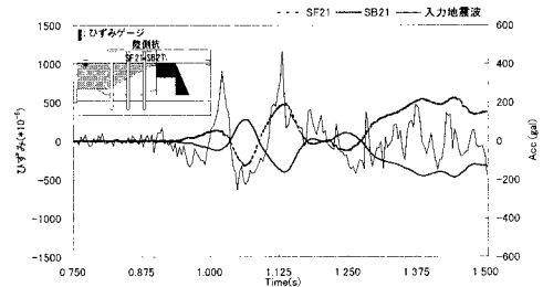
図-5 陸側杭のひずみの時刻歴 (CASE1)
