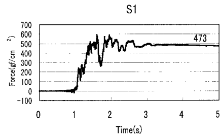
図-3 土圧の時刻歴 (S1, S2)
