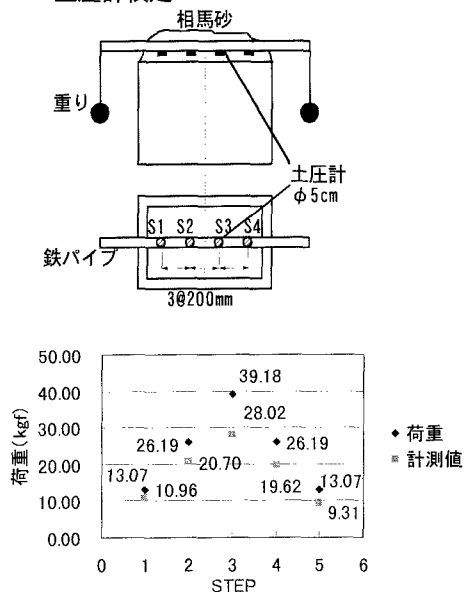
図-2 土圧計検定結果
