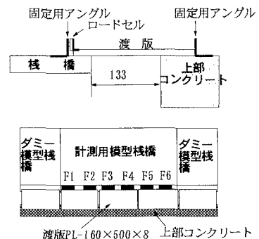
図-1 渡版および荷重計の設置方法
