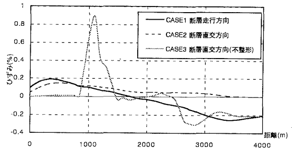
図-4 最大ひずみ発生時刻での管頂ひずみ分布図 (CASE1~CASE3)
