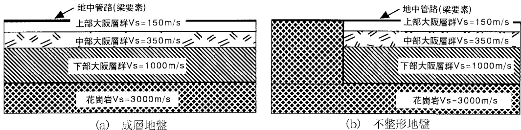
図-2 モデル図
