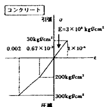
図-4 コンクリートの 非線形特性
