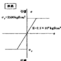
図-5 鉄筋の 非線形特性
