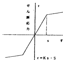
図-6 表層と 舗装版のバネ
