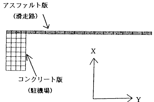
図-3 舗装版の要素モデル
