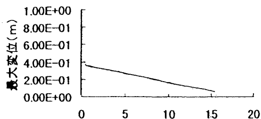
図-11 スリップバーの最大変位
