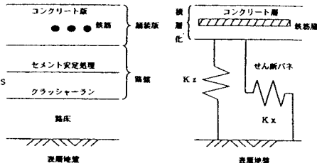
図-7 舗装版の構造と モデル図
