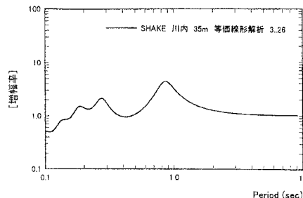
図-6 K-NET 川内における地盤の非線形を考慮した場合の伝達関数
