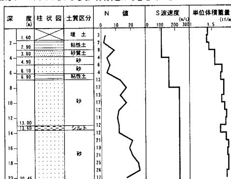
図-4 K-NET 川内の地盤構造 1)
