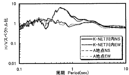
図-1 常時微動の H/V スペクトル比
