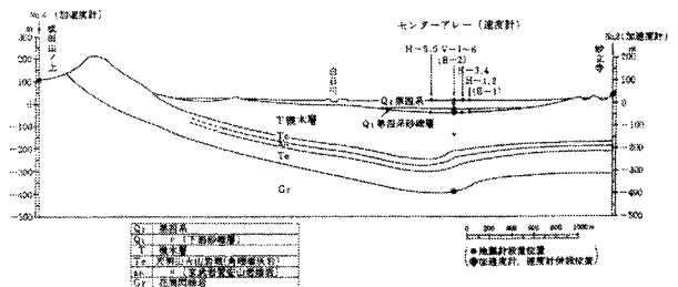
図3 地盤構造推定断面図
