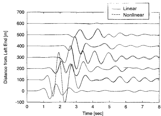
図-4 地表面における変位（鉛直成分）の時間変化
