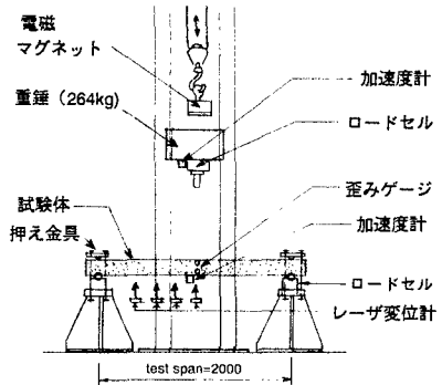
図4 試験及び計測方法
