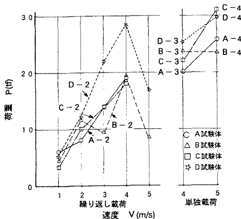
図6 速度と最大荷重の関係
