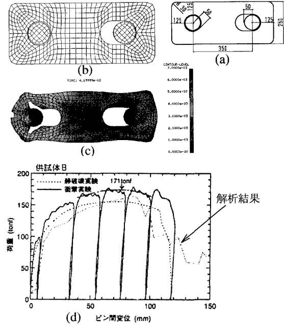
図-2 Bタイプ (矩形)
