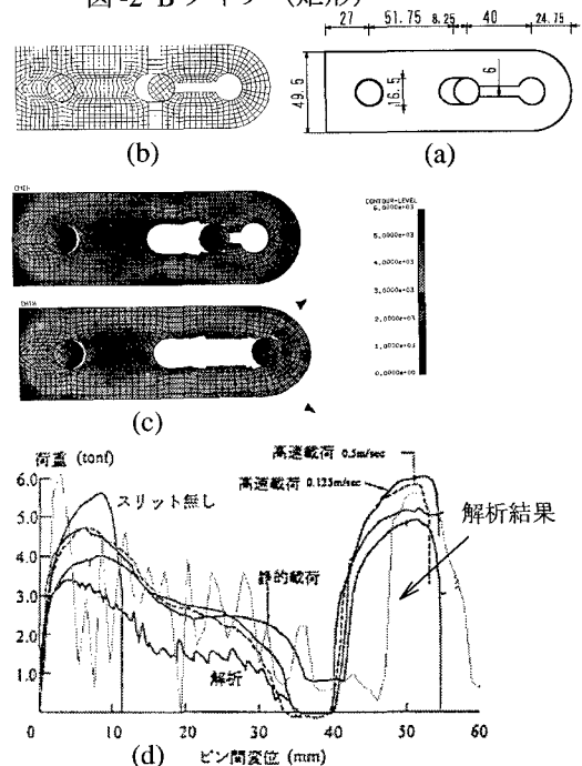
図-4 Dタイプ (スリット)
