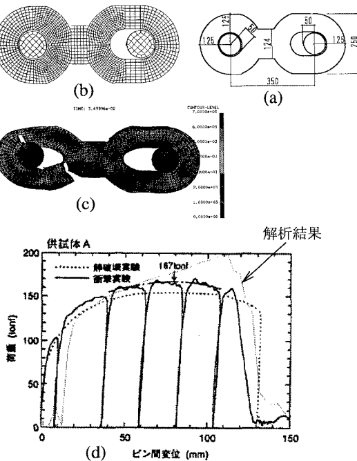
図-3 Cタイプ (アイバー)
