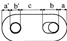
図-5 眼鏡タイプ連結板
