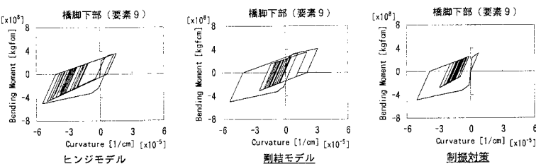
図8 橋脚基部のM- \phi 曲線
