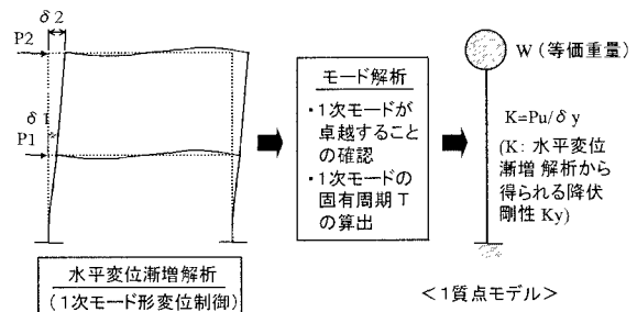
図-2 1質点系モデルへの置換
