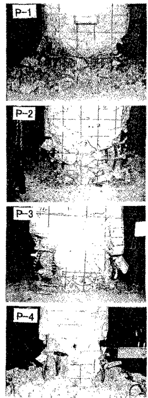
写真一1 最終損傷状況
