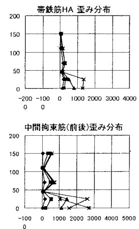
図—4 鉄筋歪（P-1）
