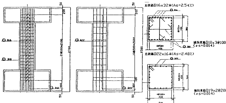
図一1 R C橋脚供試体寸法及び配筋図
