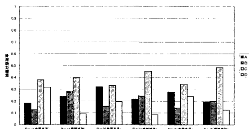
図-5 対策実施後の橋脚(橋軸方向)の損傷状態確率
