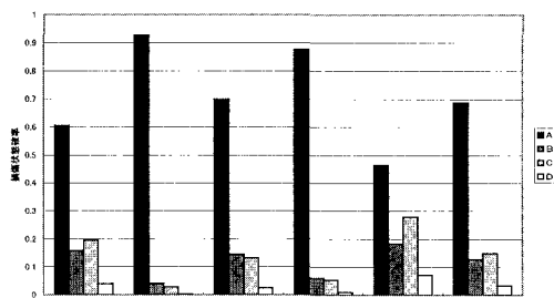
図-3 橋脚の損傷状態確率の最終値(曲げモーメント)
