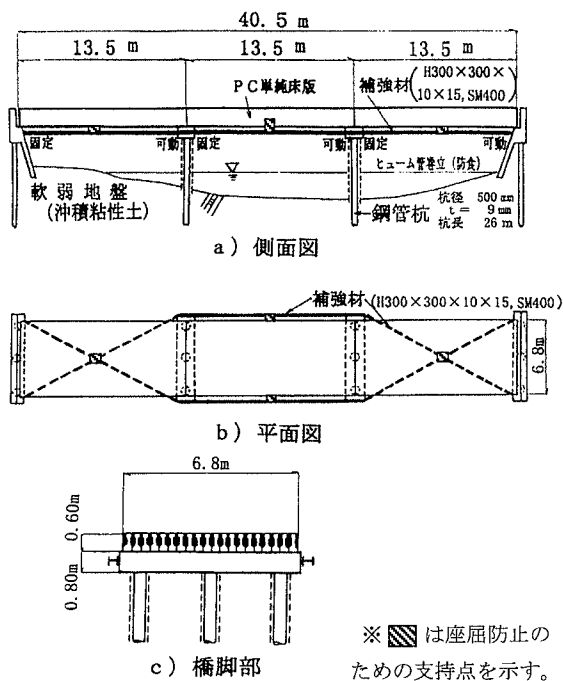
図-1 橋梁一般図
