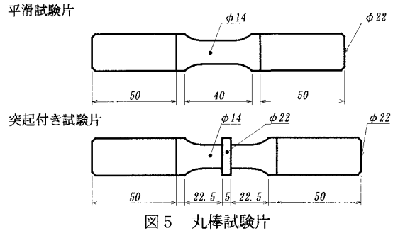
図5 丸棒試験片
