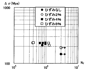
図2 リブ十字継手のS-N関係
