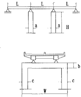
図1 対象構造モデル
