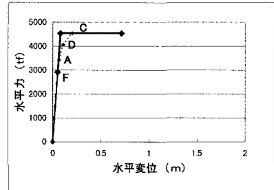
橋脚 No. 2
