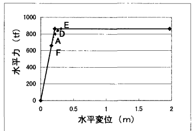
橋脚 No. 3
