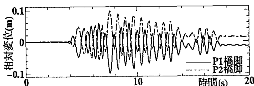
図-5-b 可動支承の相対変位時刻歴曲線
