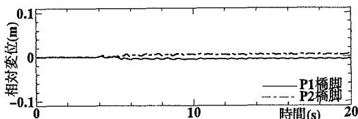
図-4-b 可動支承の相対変位時刻歴曲線
