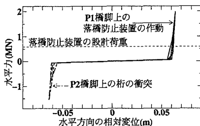
図-6-c 落橋防止装置と桁の衝突をモデル化したばねの水
