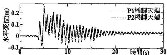
図-6-a 橋脚天端の水平変位時刻歴曲線
