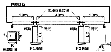
図-2 高架橋システムの解析モデル
