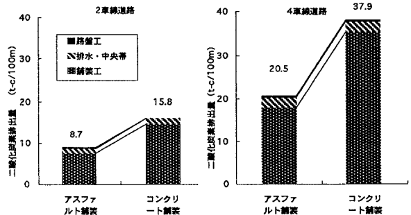
図3 幅員別 CO 2 排出量
