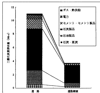
図2 産業部門別CO 2 排出量
