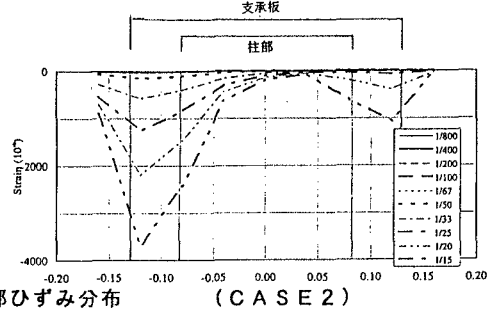
図-6 基礎部ひずみ分布
