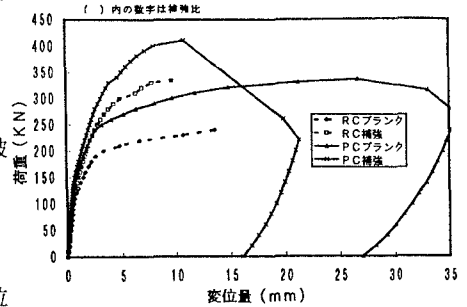
図1 ボックスカルバートの荷重-変位曲線 (上辺と下辺の間の距離)
