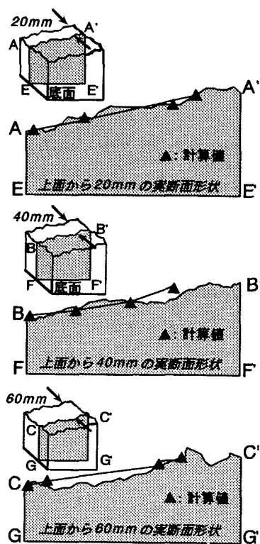
図-4 実測値と計算値との比較
