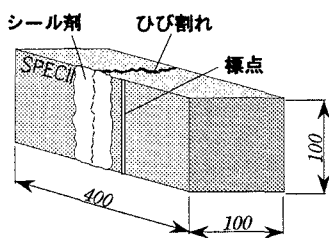
図-2 ひび割れ形状検出用供試体
