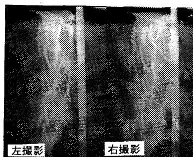
写真-1 X線フィルムより 検出されたひび割れ
