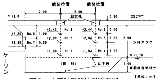
図3 土圧計設置位置断面図
