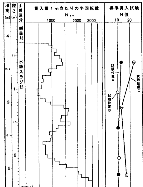
図4 標準貫入試験およびスクエーデン式サウンディング試験の結果
