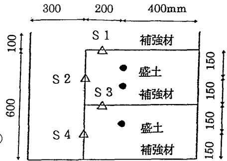
図-1 実験装置 ●：加速度計 △：ひずみゲージ
