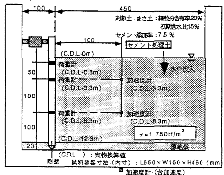
図-2 遠心模型地盤概要
