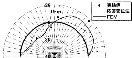
図 2 曲げモーメント図
