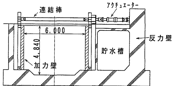
図-1 大型せん断土槽断面
