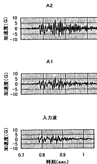
図-3 応答加速度時刻歴
