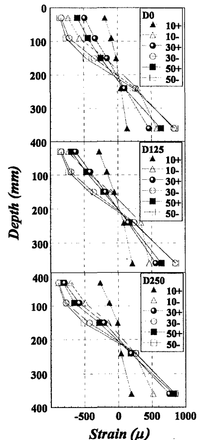
図-4 曲げ歪の分布
