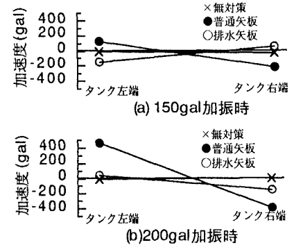
図-4 タンク両端の鉛直加速度
