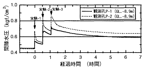
図－5 間隙水圧測定結果
