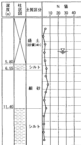
図－1 地盤条件
