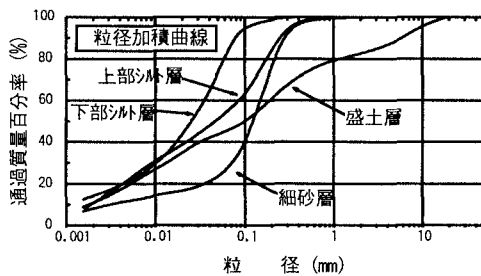
図－2 粒度分布
