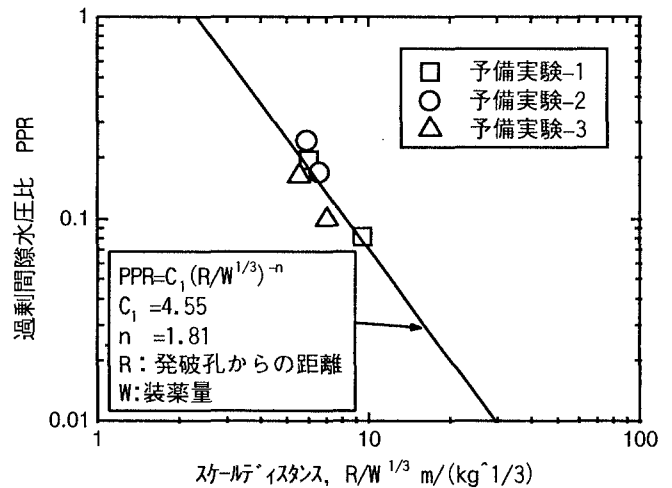
図－6 間隙水圧ースケールディスタンス関係
