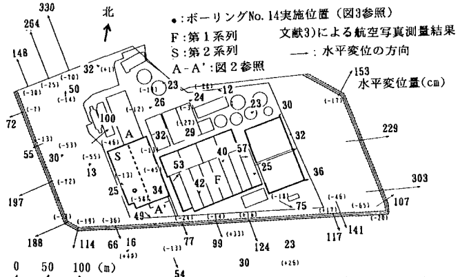
図1 西部処理場の平面図
