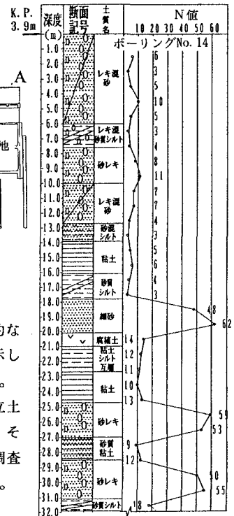
図3 地震前の地盤調査結果の例
