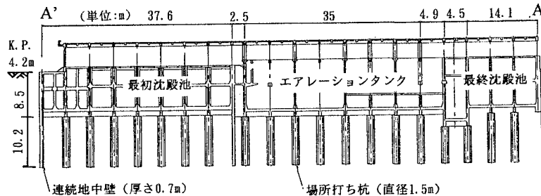
図2 第2系列污水处理施設の代表的断面図
