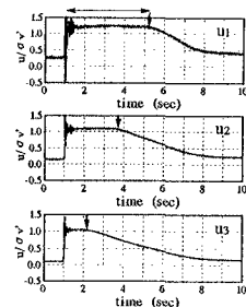
図-3 過剰間隙水圧比時刻歴
