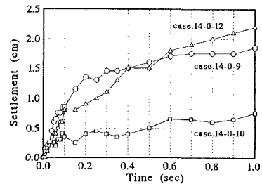
図-2 時間的な模型盛土の沈下
