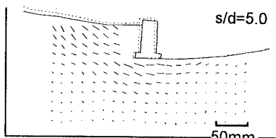
図3 地盤の残留変位ベクトル
