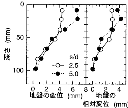
図7 地盤の残留変位と杭との相対残留変位
