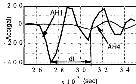
図-3 板たたき法による初期 せん断波速度の計測
