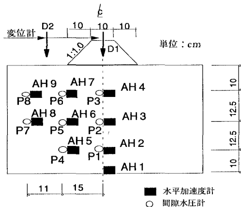
図-1 実験土層
