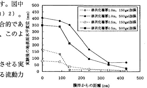
図-5 護岸からの距離と地表面水平変位の関係
