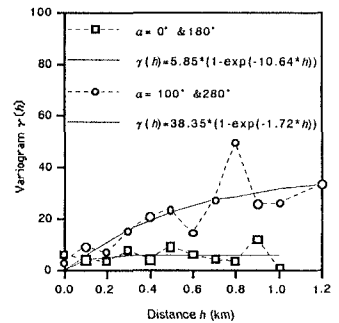
図5 バリオグラム
