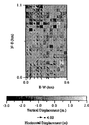
図1 対象地区の地盤変位
