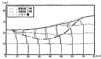
図-6 振動終了後の変位量 (CASE II)
