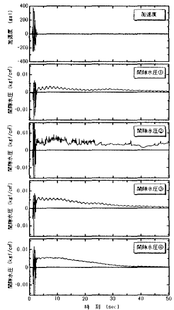
図-9 加速度と間隙水圧の時刻歴
