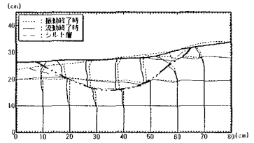
図-8 振動終了後の変位量 (CASE III)
