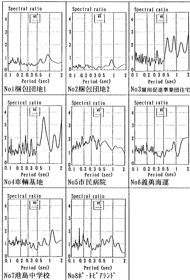
図-1 六甲アイランドのH/Vスペクトル比
