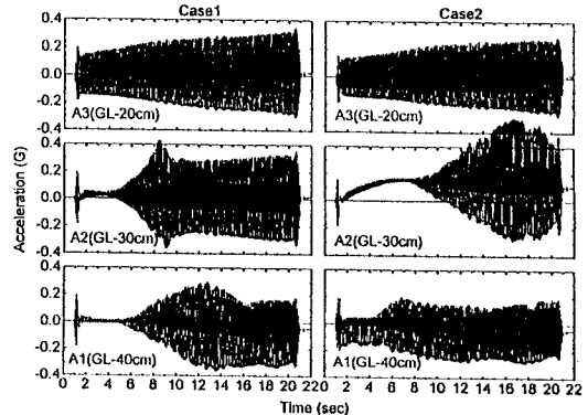
図-6 加速度計の経時変化図（基礎直下）
