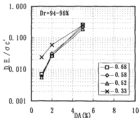
図 2 繰返し非排水三軸試験結果
