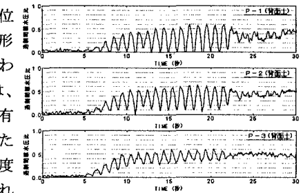
図-5; 裏込め石のない場合の過剰間隙水圧比の時刻歴応答
