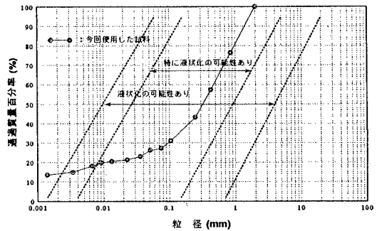
図-1 ; 粒度分布 (港湾の基準を盛り込んだもの)
