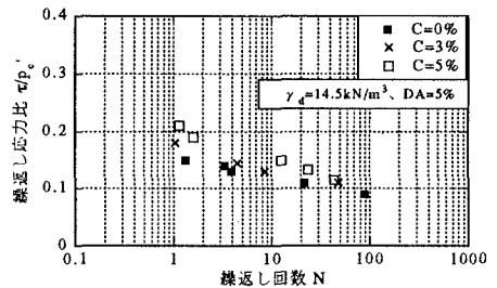
図-5 液状化強度曲線
