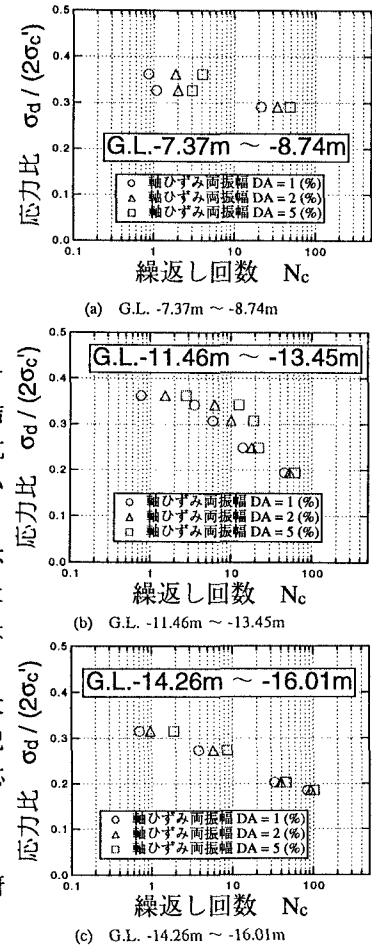
図3 液状化試験結果
