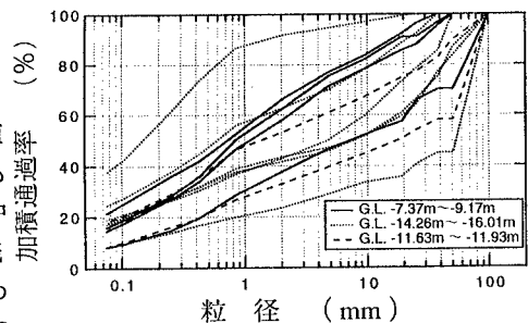
図2 凍結サンプリング試料の粒度分布
