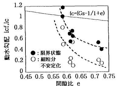
図5 e と l_{cf}, l_c
